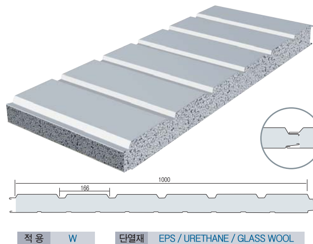
R.P 5골 노몰드
