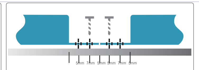
시공순서 3 - 매지간격 34m/m 시공 (m 2 / 4.29장)
