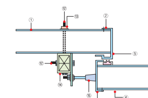
하부스토바 구성도
