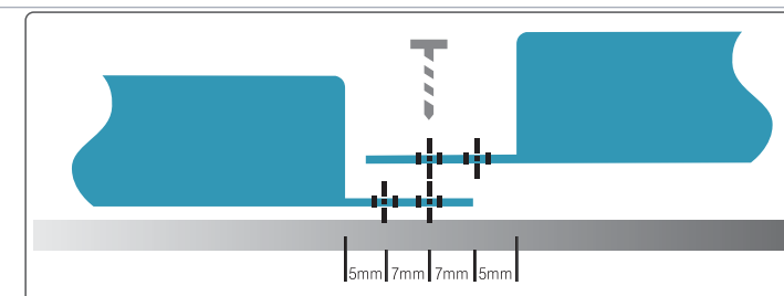
시공순서 2 - 매지간격 24m/m 시공 (m 2 / 4.45장)
