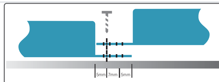
시공순서 1 - 매지간격 17m/m 시공 (m 2 / 4.58장)
