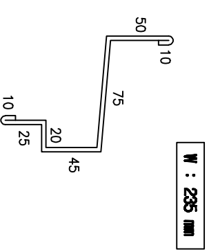
C/S 0.5T 마감 FLASHING
