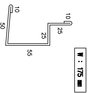
C/S 0.5T 마감 FLASHING
